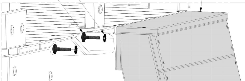
407 (x2) BOULON - 1 1/2"
